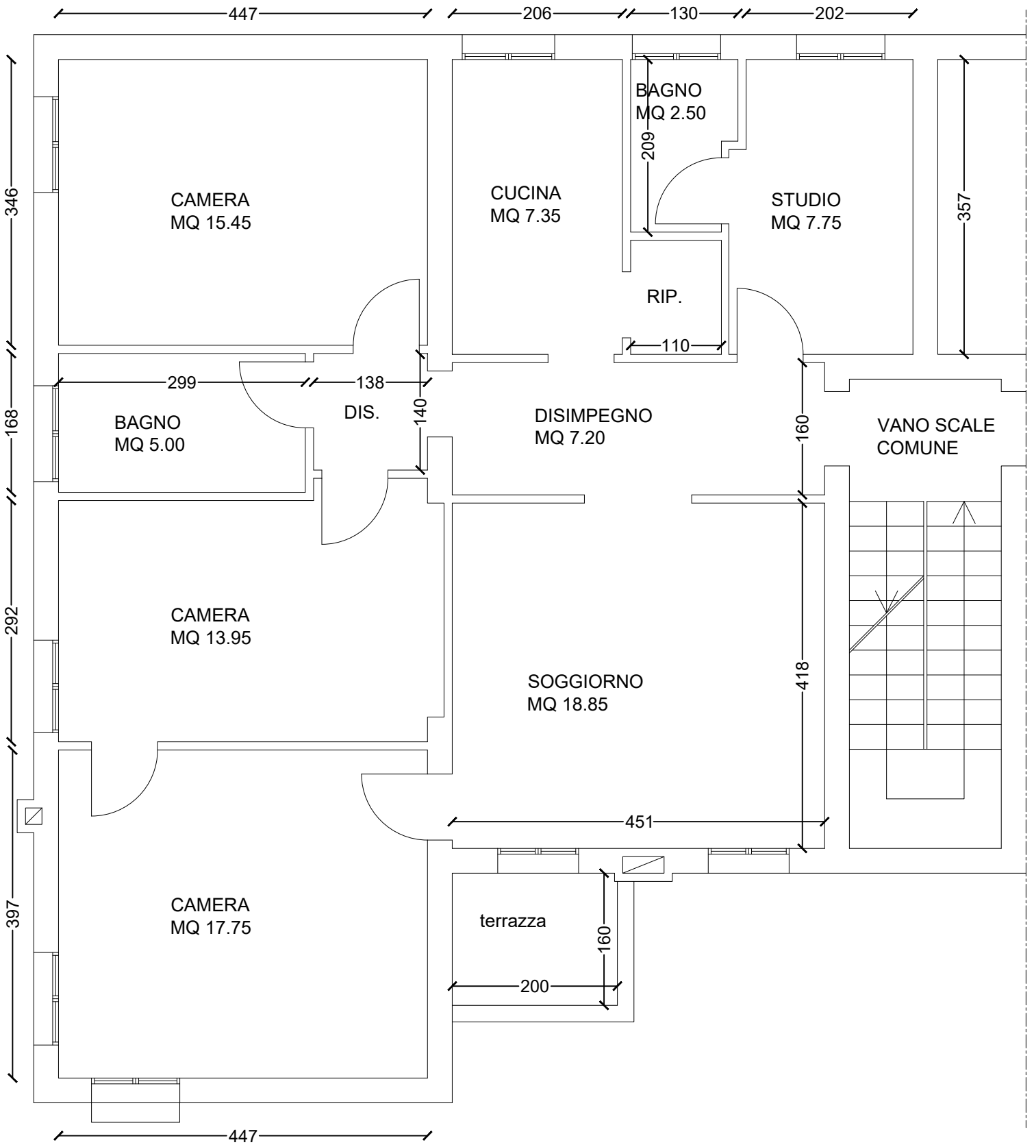
PIANTA PIANO SECONDO STATO DI FATTO
